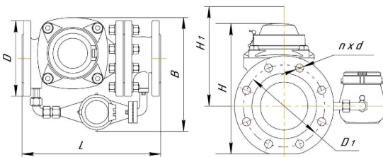
Рис. 2 Размеры счетчика CTBK 2
